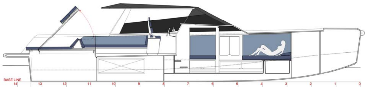
Longitudinal Section
